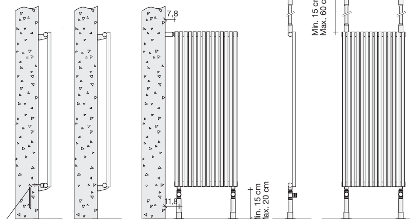
Allacciamento al Gruppo Valvole Remoto (GVR) con attacco B2R Supporto STANDARD A MURO (cod. ST)
