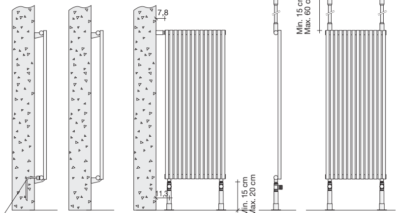
Supporto STANDARD A MURO (cod. ST)
