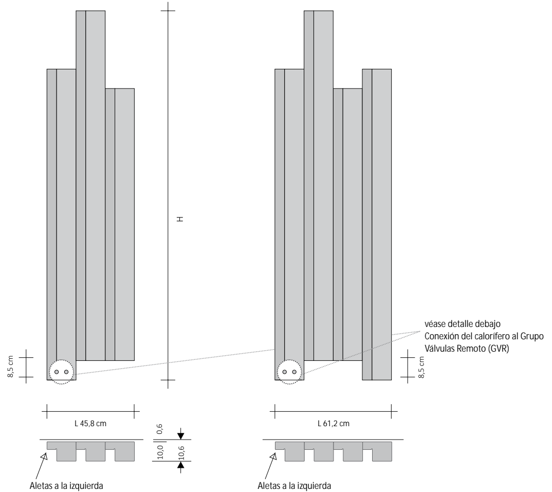
Conexión del GVR
