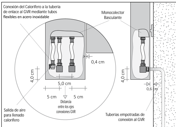
Conexión del calorífero al Grupo Válvulas Remoto (GVR)
