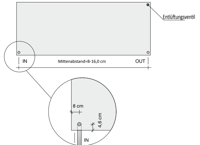
Anschluss des HEIZKÖRPERS an GVR
