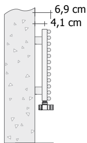
Support STANDARD MURAL (réf. ST)
