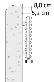
Support STANDARD MURAL (réf. ST)
