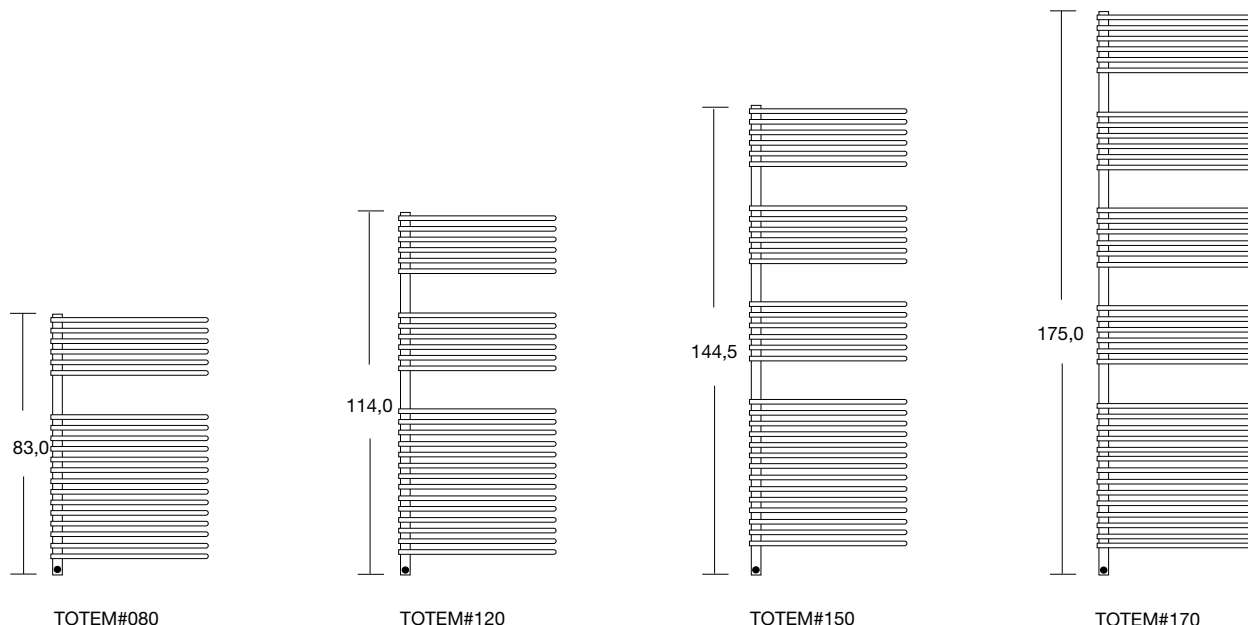
Distancia entre ejes de las conexiones con medidas referidas a las válvulas Tubes
