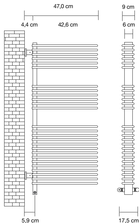
Distancia entre ejes de las conexiones con medidas referidas a las válvulas Tubes
