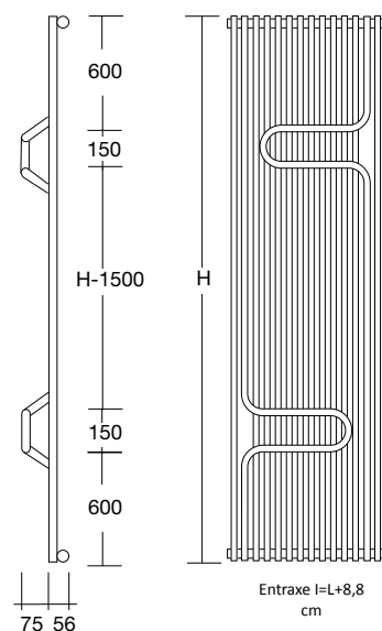
AK2 - VERSION HYDRAULIQUE STANDARD DOUBLE POIGNÉE (raccords OC1)
