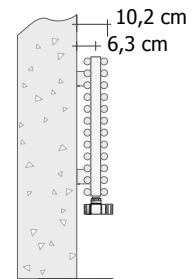
WAND-STANDARDHALTERUNG (Code ST)
