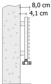
WAND-STANDARDHALTERUNG (Code ST)
