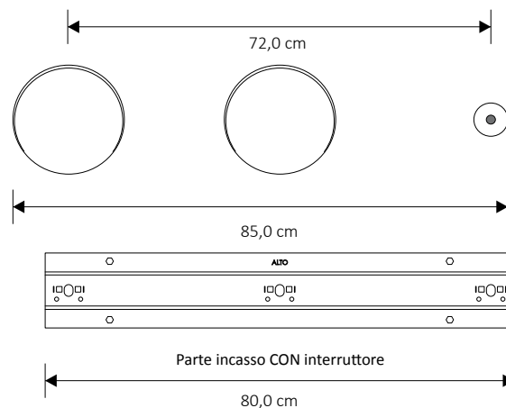
Versione CON interruttore
