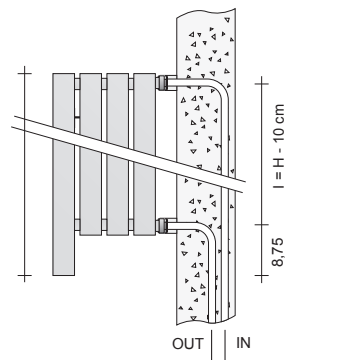
Anschluss an die Ventilgruppe mit Remote-Anschluss (GVR)
